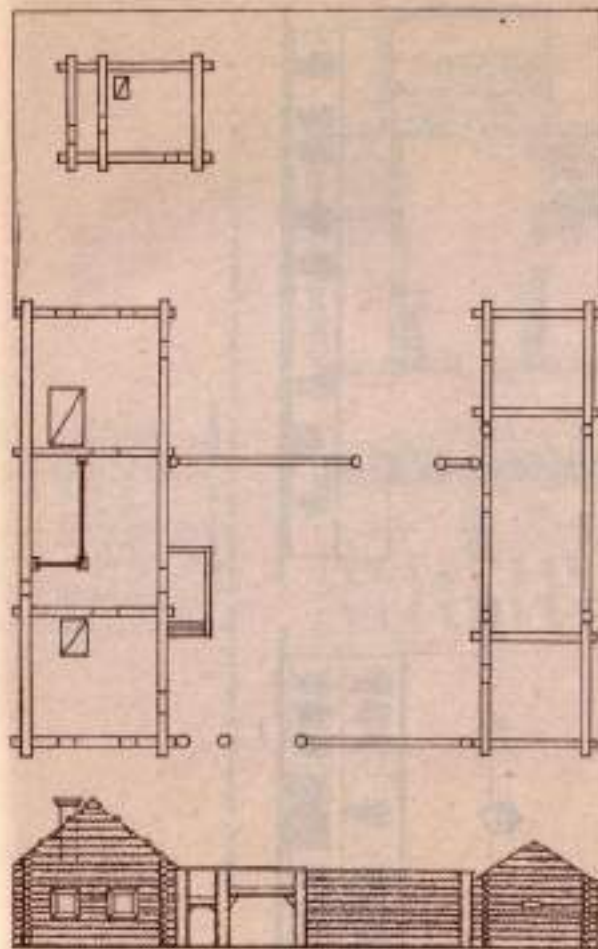
План и фасады крестьянской усадьбы конца XVIII в. Кольчано-Воскресенского Горного округа. Публикуется впервые.
